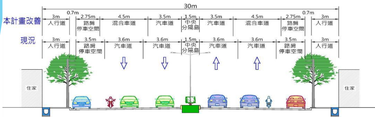
鹿峰國小旁中山路改善前後車道斷面圖
